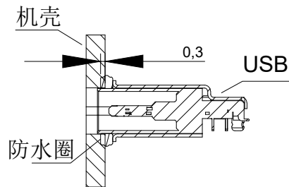
组装示意图
