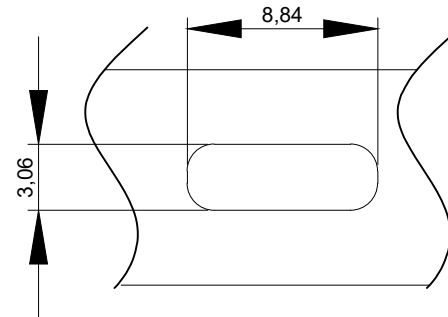
机壳尺寸图
