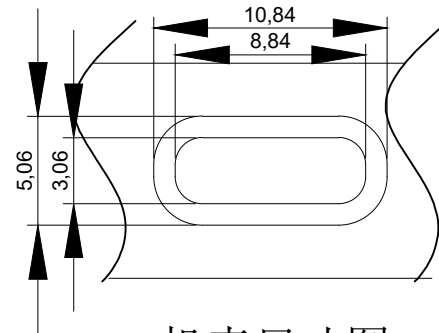
机壳尺寸图
