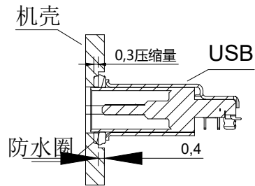
组装示意图
