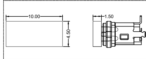
CAP DIMENSIONS
