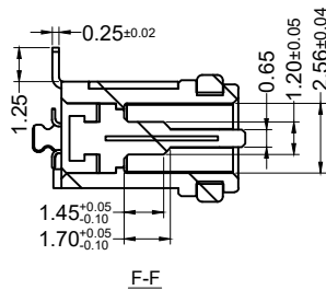
CAP DIMENSIONS
