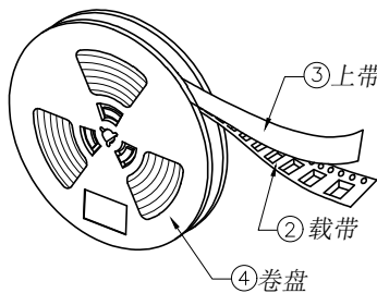
卷盘示意图
