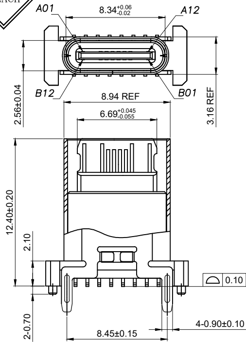
剖视图
