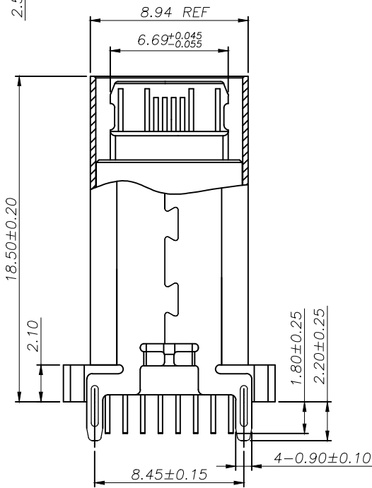
剖视图
