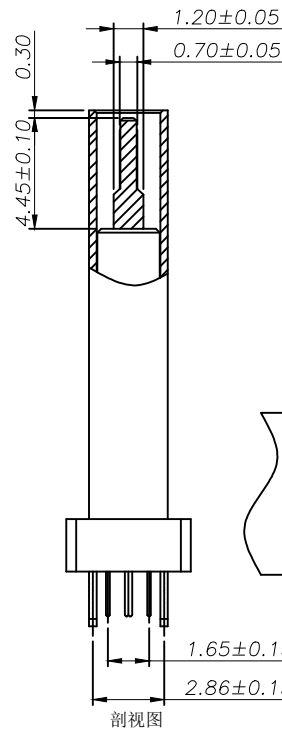
剖视图
